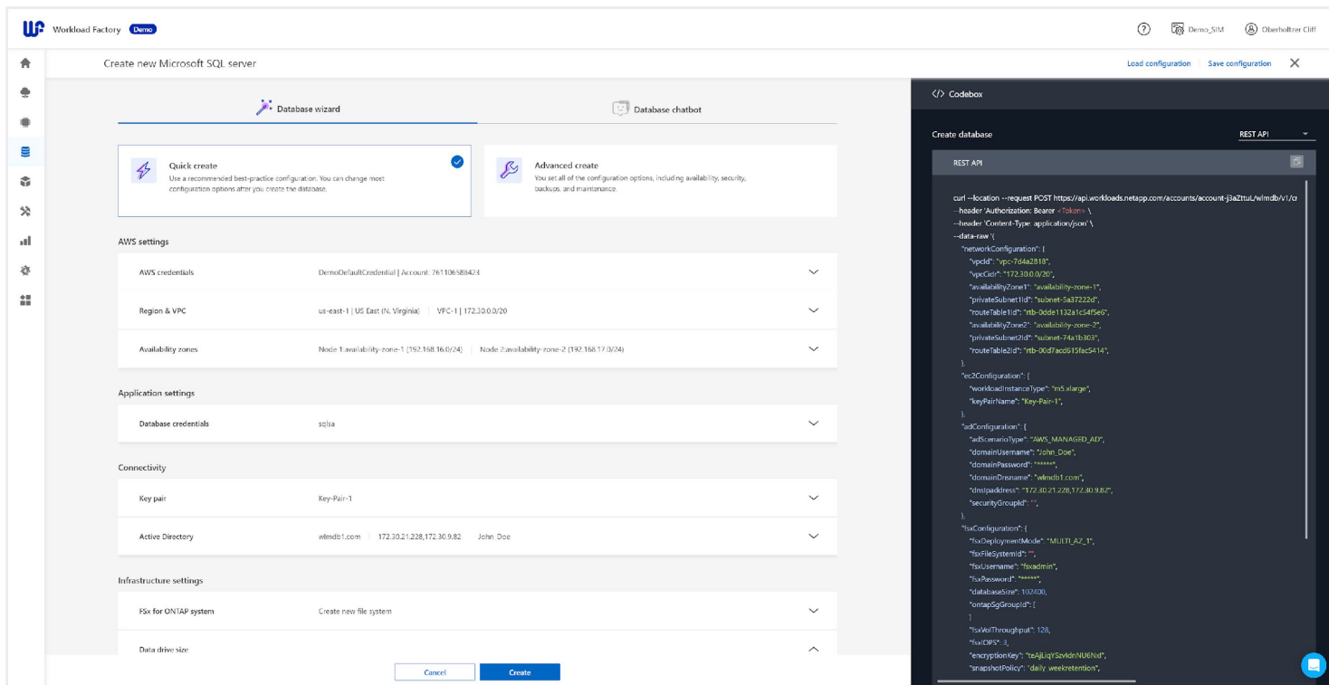
圖 3：建立資料庫。
