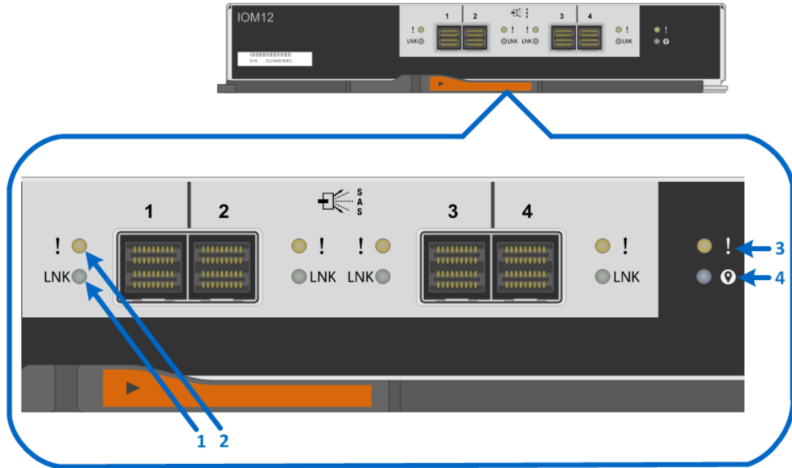
Figure 52) LEDs for IOM.
