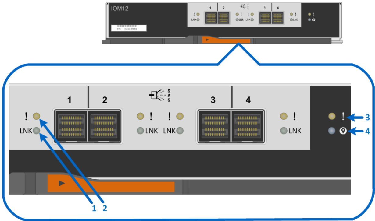
Figure 45) LEDs for IOM.
