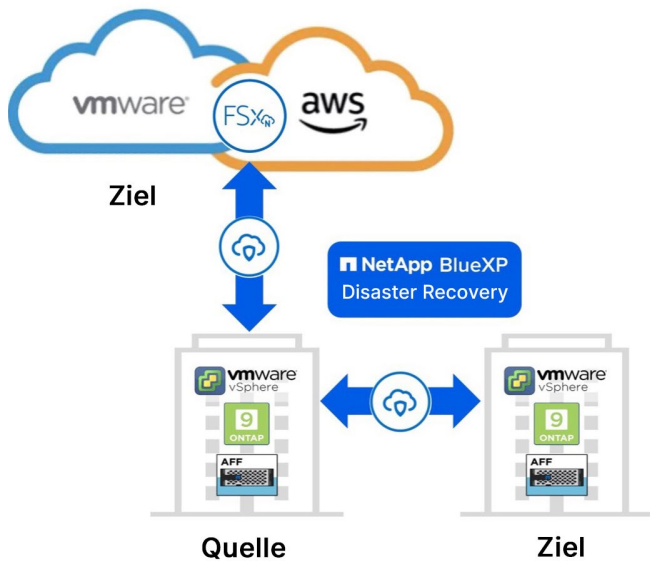
Abbildung 1: Zur Disaster Recovery mit BlueXP können Sie eine ONTAP On-Premises-Umgebung oder VMware Cloud oder Amazon FSx for NetApp ONTAP nutzen.
