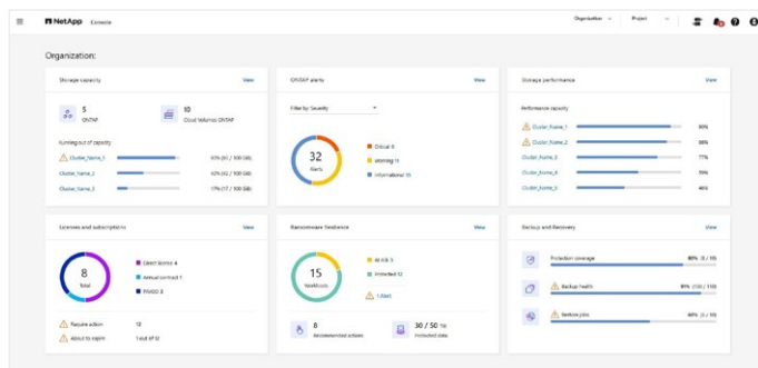
Abbildung 1: NetApp -Konsole
